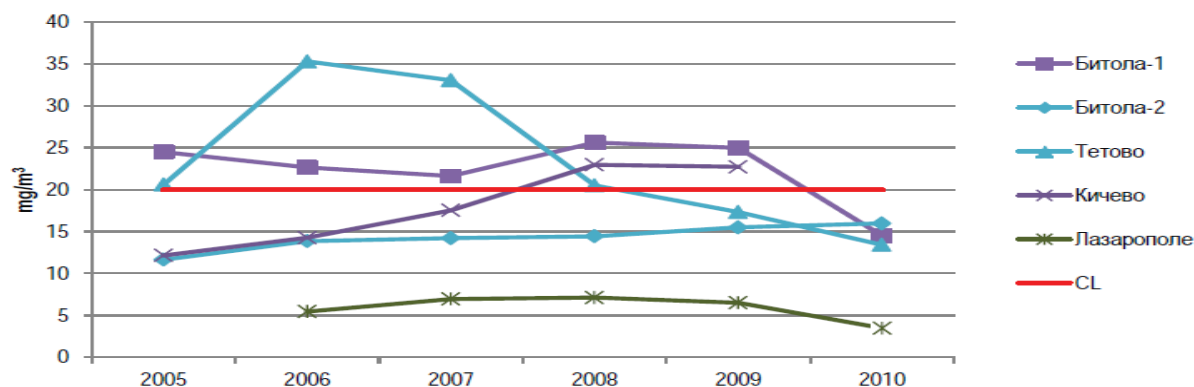
Графикон бр. 3. Просечни годишни концентрации на сулфур диоксид во Западна зона за период 2005- 2010 година
